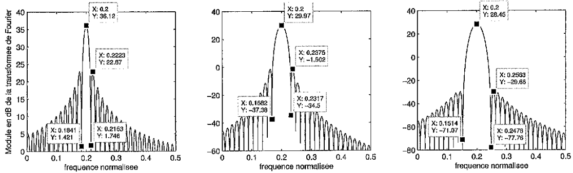
FIGURE 1 – Transformée de Fourier à temps discret à l'aide de 3 fenêtres
